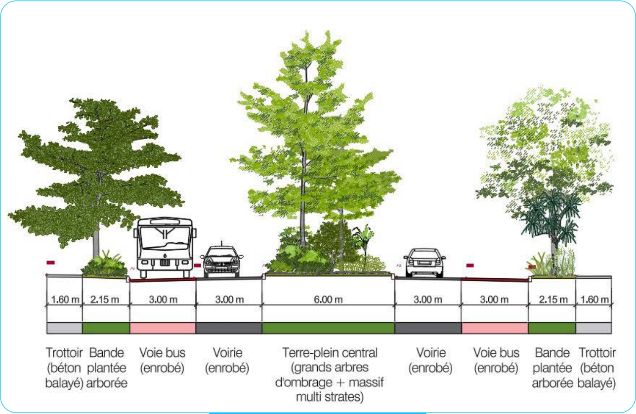
Coupe Projet rue Hélène Boucher
