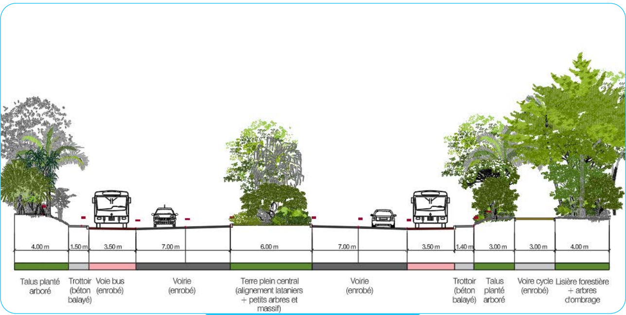
Coupe Projet tronçon RN102
